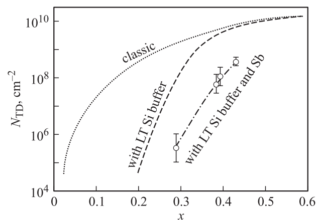
Рис. 3. Плотность пронизывающих дислокаций N_{TD} в пластически релаксированных пленках \text{Ge}_x\text{Si}_{1-x} ступенчато изменяемого состава, выращенных с использованием сурфактанта Sb (точки и штрих-пунктирная линия), в сравнении с обобщенными данными рис. 1 (пунктирная и штриховая линии).
